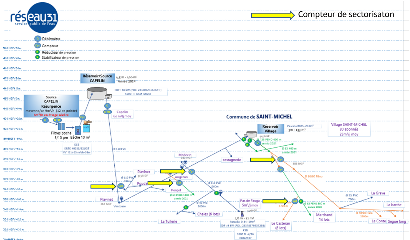
Synoptique du réseau de distribution de la commune de Saint-Michel – données Réseau31
