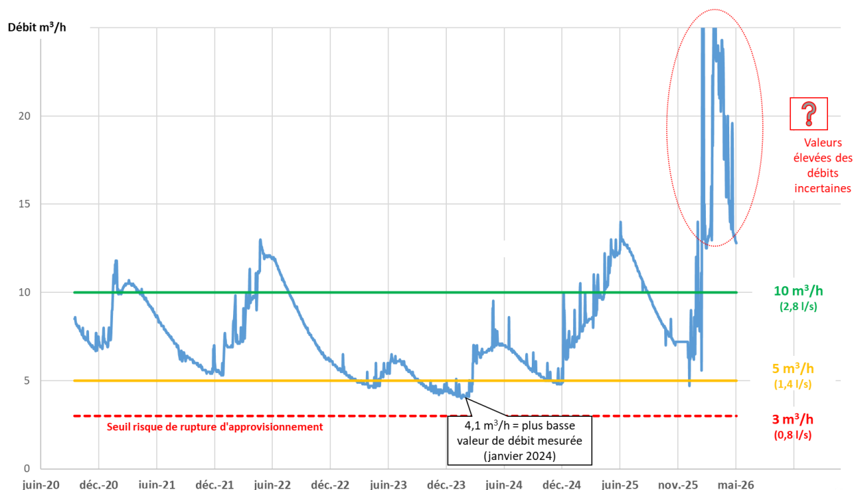
Evolution du débit de la source de Capelin (2020 – 2026) – données Réseau31
